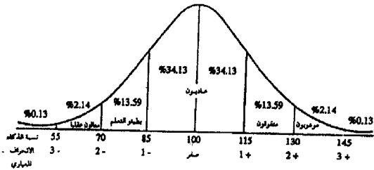
منحنى التوزيع الطبيعي للقدرة العقلية
